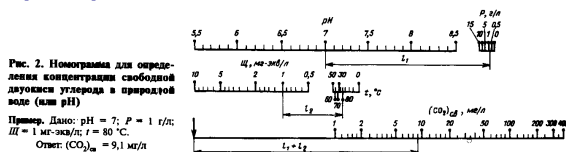
"Рис.2. Номограмма для определения концентрации свободной двуокиси углерода в природной воде (или \text{pH} )"
